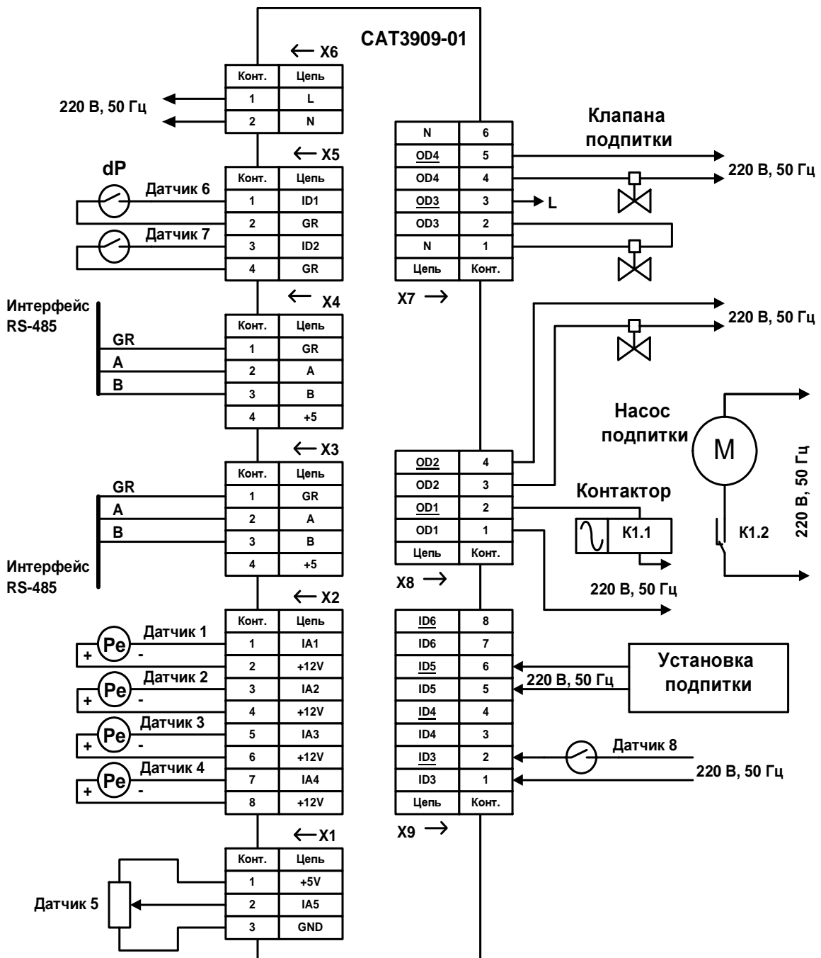
Рисунок 6 - Электрическая принципиальная схема подключения CAT3909-01 (типовая)
