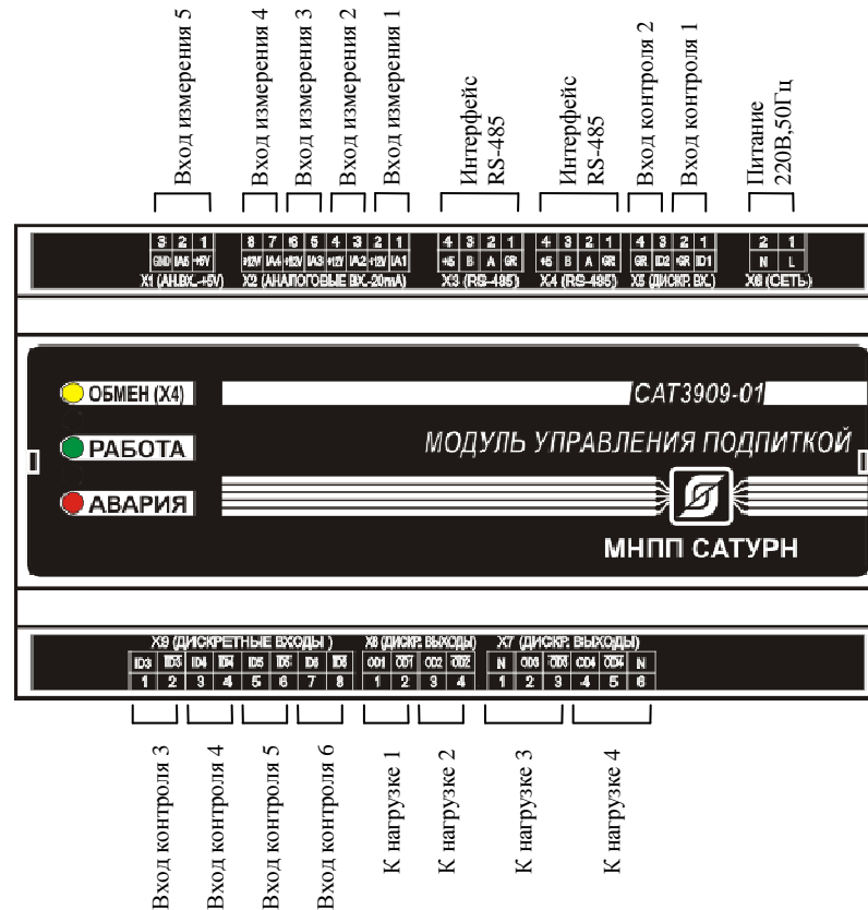
Рисунок 5 - Расположение разъёмов на модуле САТ3909-01
