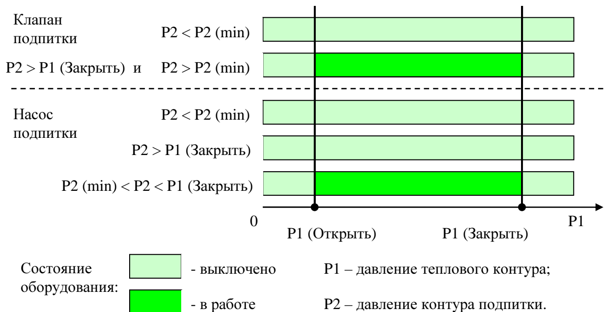
Рисунок 2 - Диаграмма работы узла подпитки
