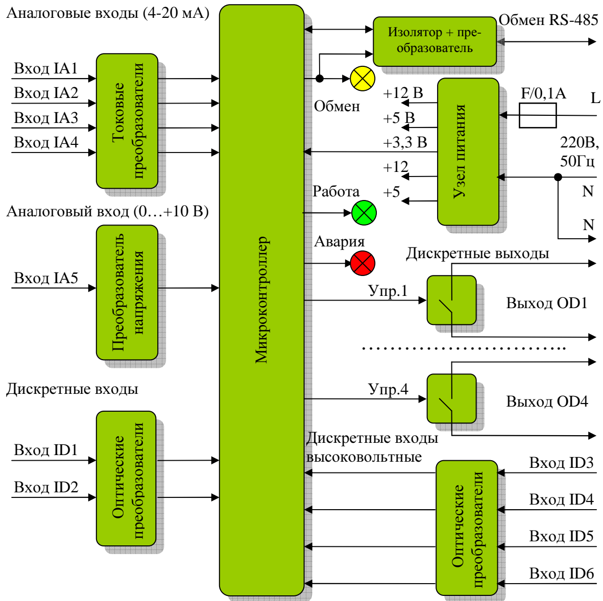
Рисунок 3 - Структурная схема САТ3909-01
